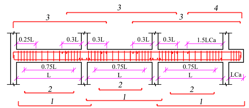
شكل نموذجي لتوزيع حديد التسليح في الكمرات
